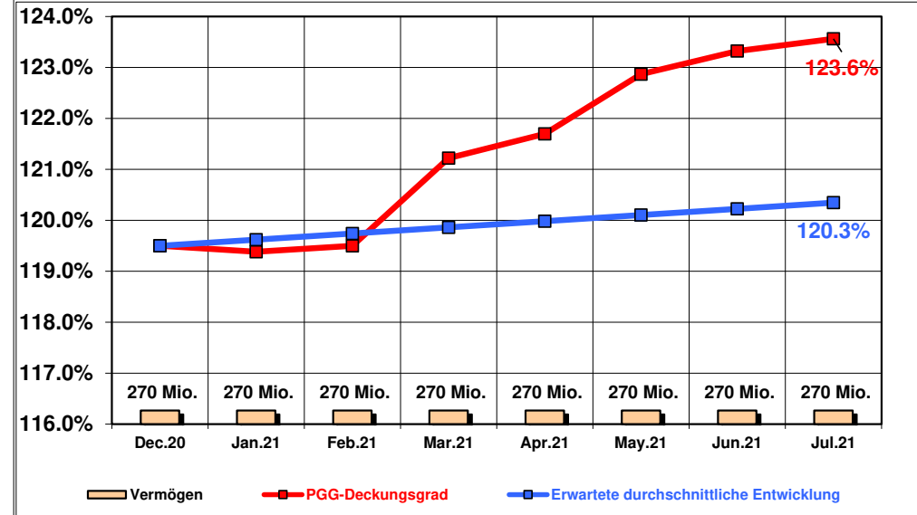
Geschätzte Deckungsgradentwicklung
